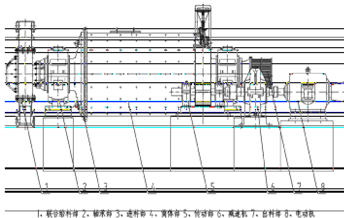
1. 联合给料器 2. 轴承座 3. 进料器 4. 筒体 5. 传动部 6. 减速机 7. 出料器 8. 电动机
